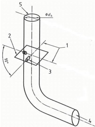
1-采样线；2-采样平面；3-采样孔（法兰）；4-流动方向；5-烟道顶端
